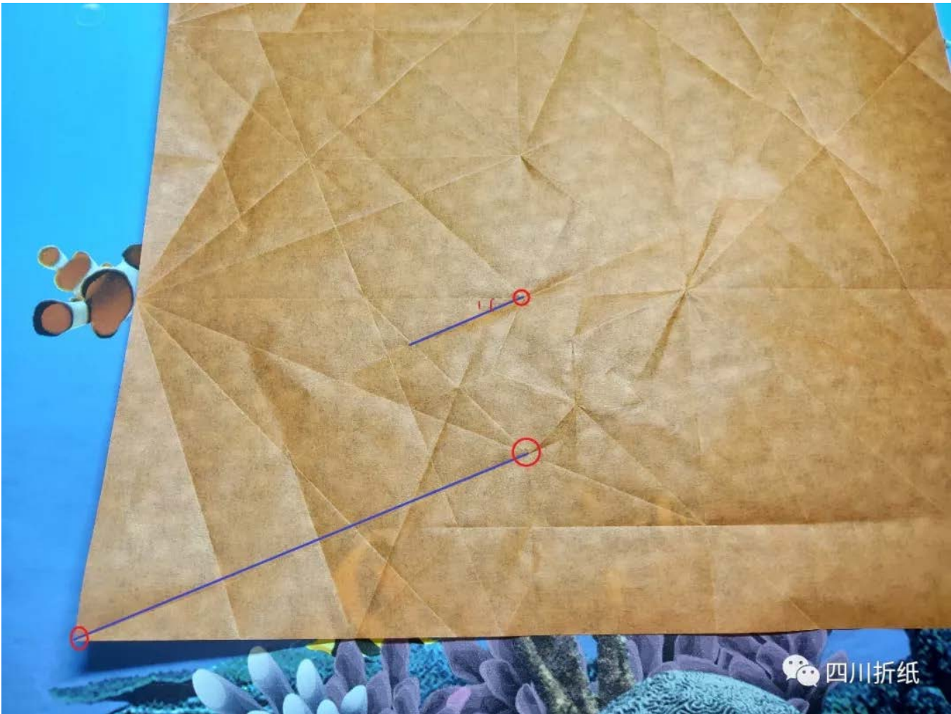
作出垂线
