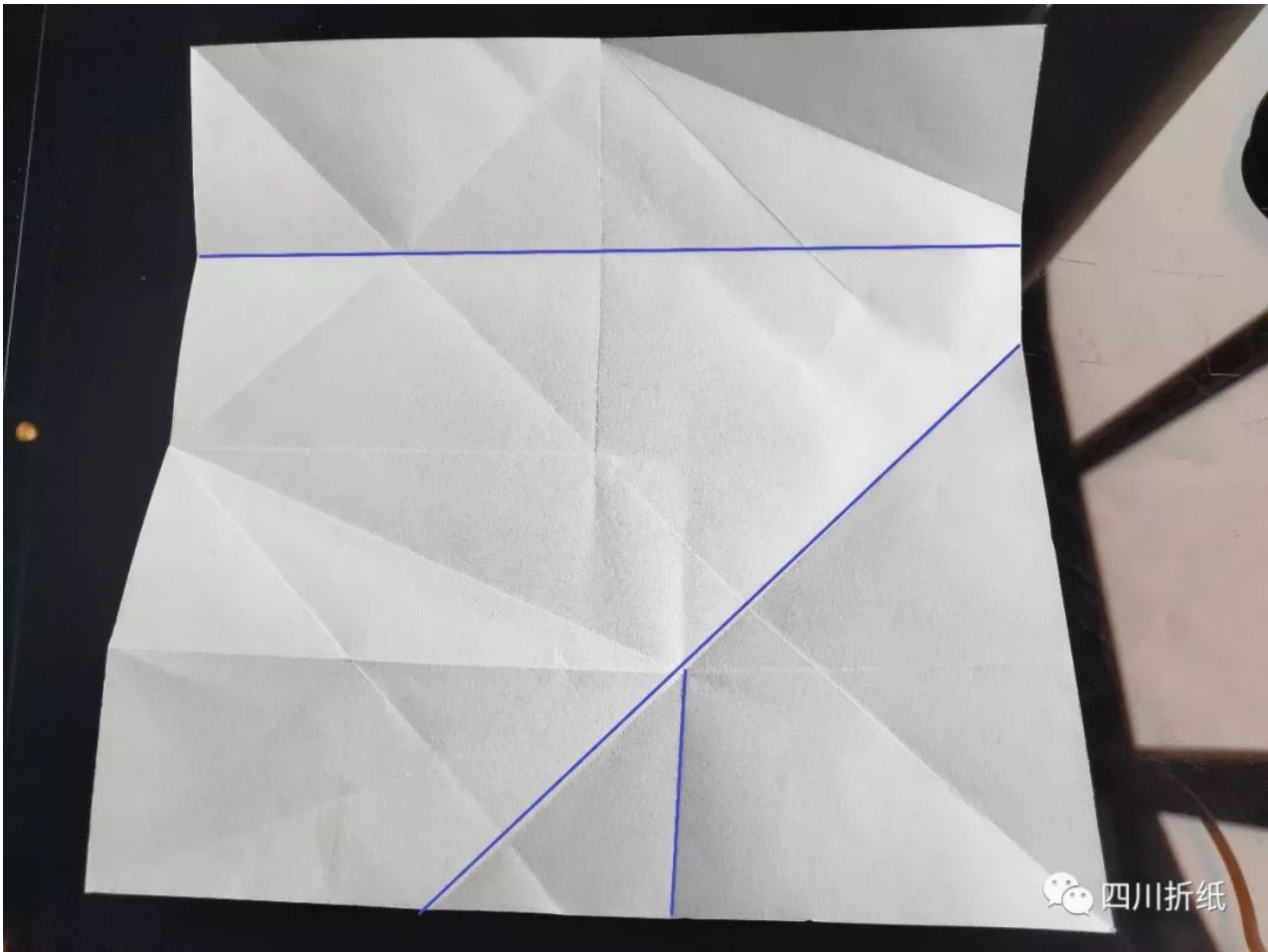
3为12角平分线
